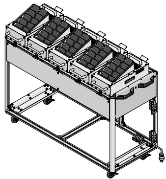
アイソメビュー (1:20)
