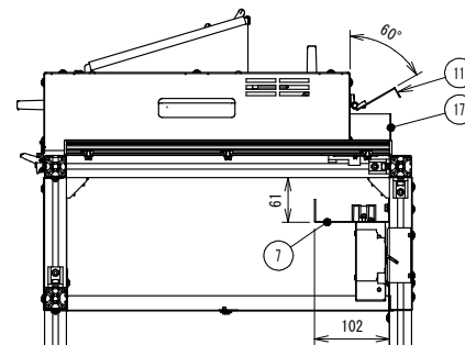
断面図 A-A (1:8)
