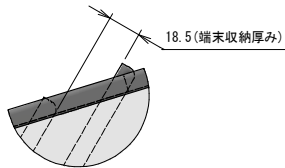
詳細図 B (1 : 3)
