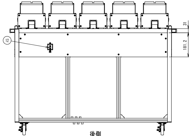
後側
