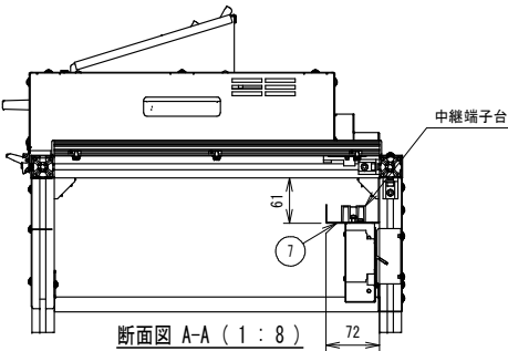
断面図 A-A (1 : 8)
