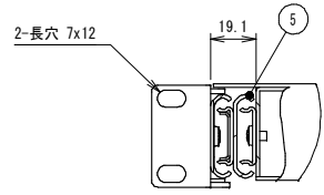
詳細図 A (1:2.5) (左右同様)
