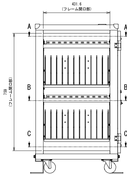
右扉開き時 ( 1 : 10 )
