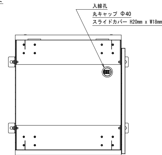
断面図 C-C ( 1 : 8 ) (底部詳細)
