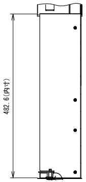
断面図 B-B (1:8)
