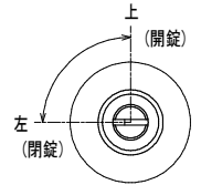
P部 詳細図 (1:2) (左位置のみ鍵の抜き差しが可能)
