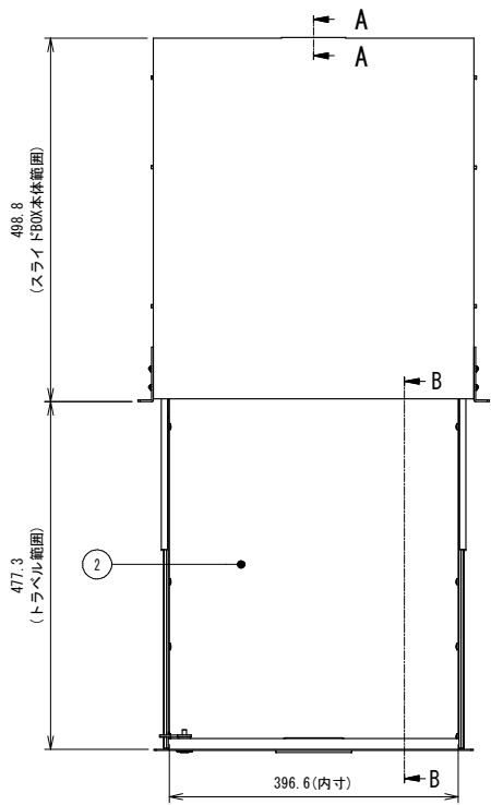
平面図 (1:8) (BOX引出時)
