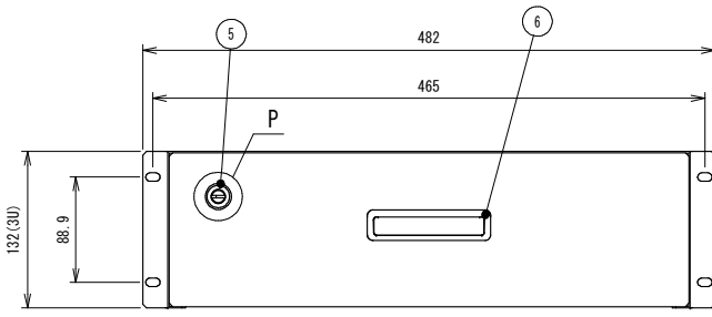
正面図
