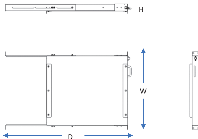
外観図
